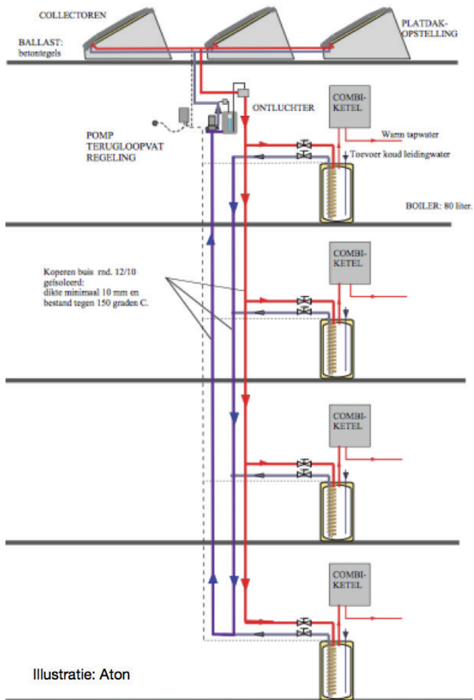
Schema Aton hoogbouwsysteem
